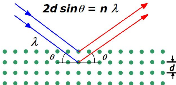
Slika 4.1: Braggov uklon je uklon oziroma sipanje rentgenskih žarkov na kristalni mreži. Pri tem pride v določenih smereh zaradi interference do močnih ojačanj. Slika je povzeta iz [13].
