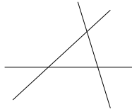
SLIKA 6. Ncentralna razporeditev s sedmimi centralnimi podrazporeditvami.
