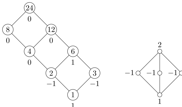
SLIKA 5. Hassejev diagram in vrednosti Möbiusove funkcije za D_{24} in za L(\mathcal{B}_3) .
